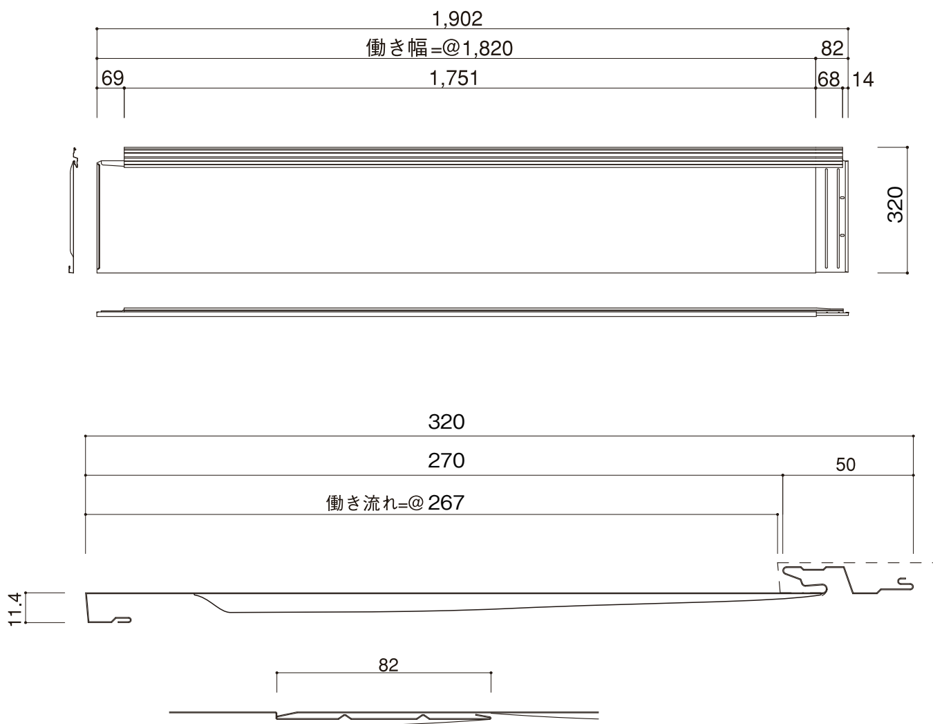
ヨコ連結部詳細（断面）
