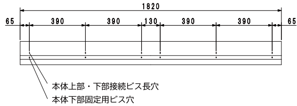
2P本体側面図 (2P=1820)
