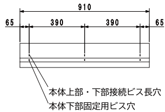
1P本体側面図 (1P=910)
